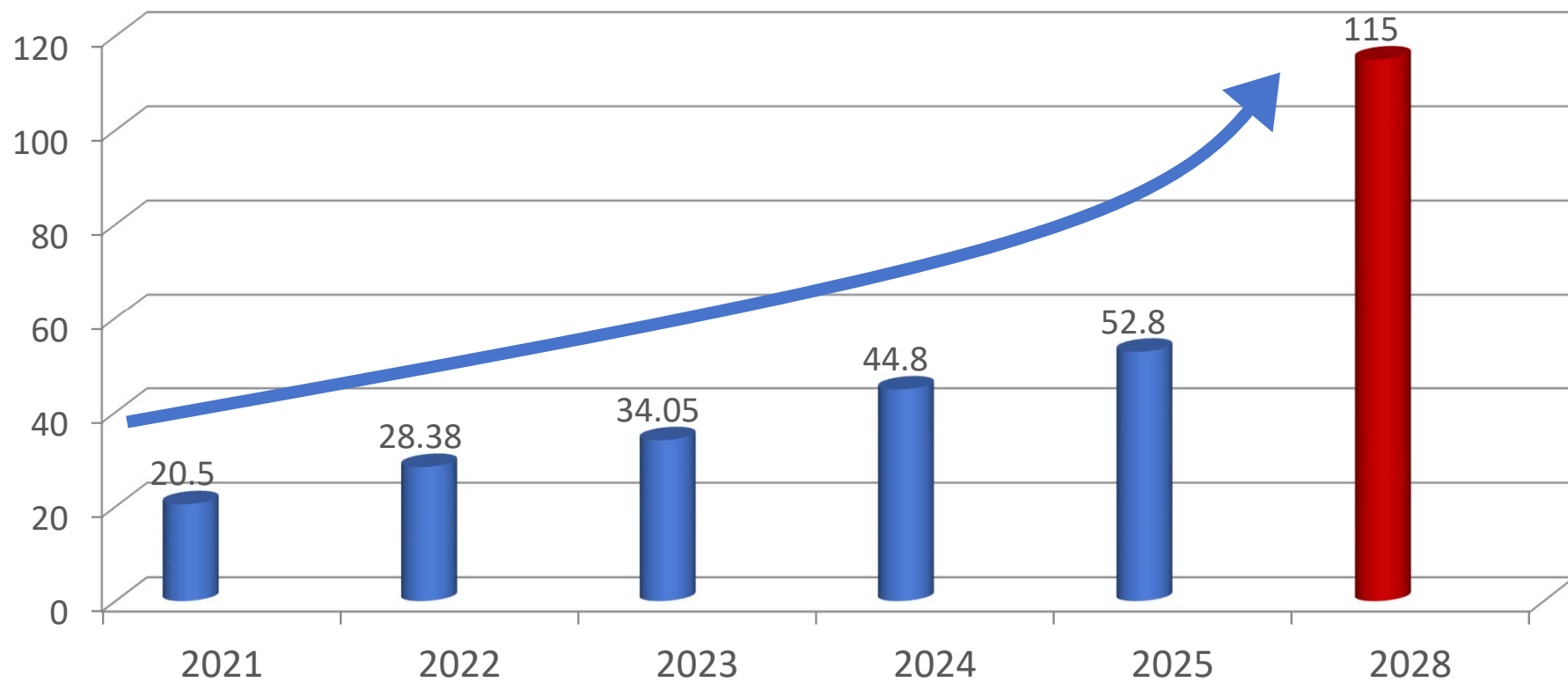
Tag IC Volume (Billion)
